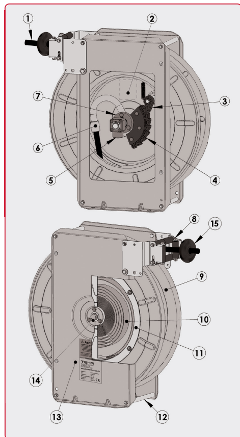
Abb. 1 - Schlauchaufroller
