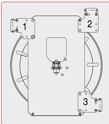
Abb. 2 - Varianten Schlaucheinlauffenster
