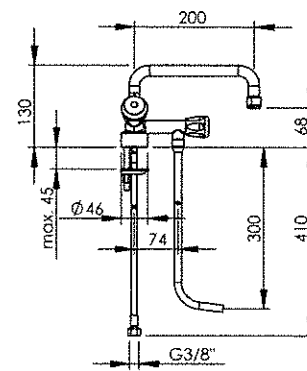
Maßzeichnung 100.101 C
